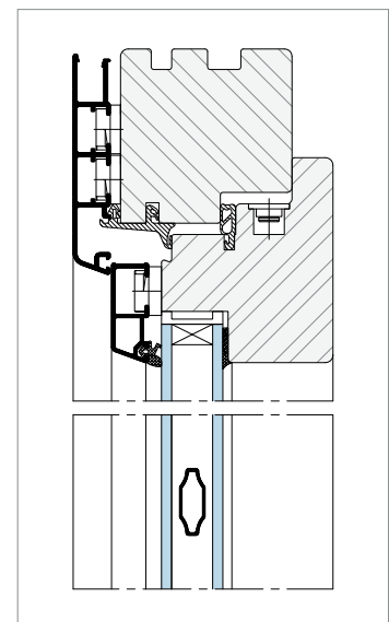
Sprosse im Scheiben- zwischenraum
