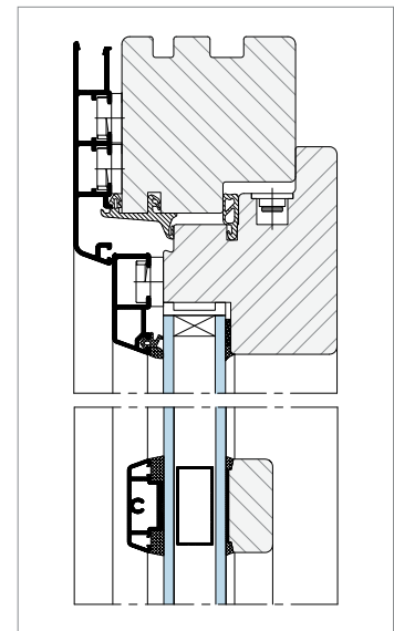
Aufgesiegelte Sprossen 36 mm
