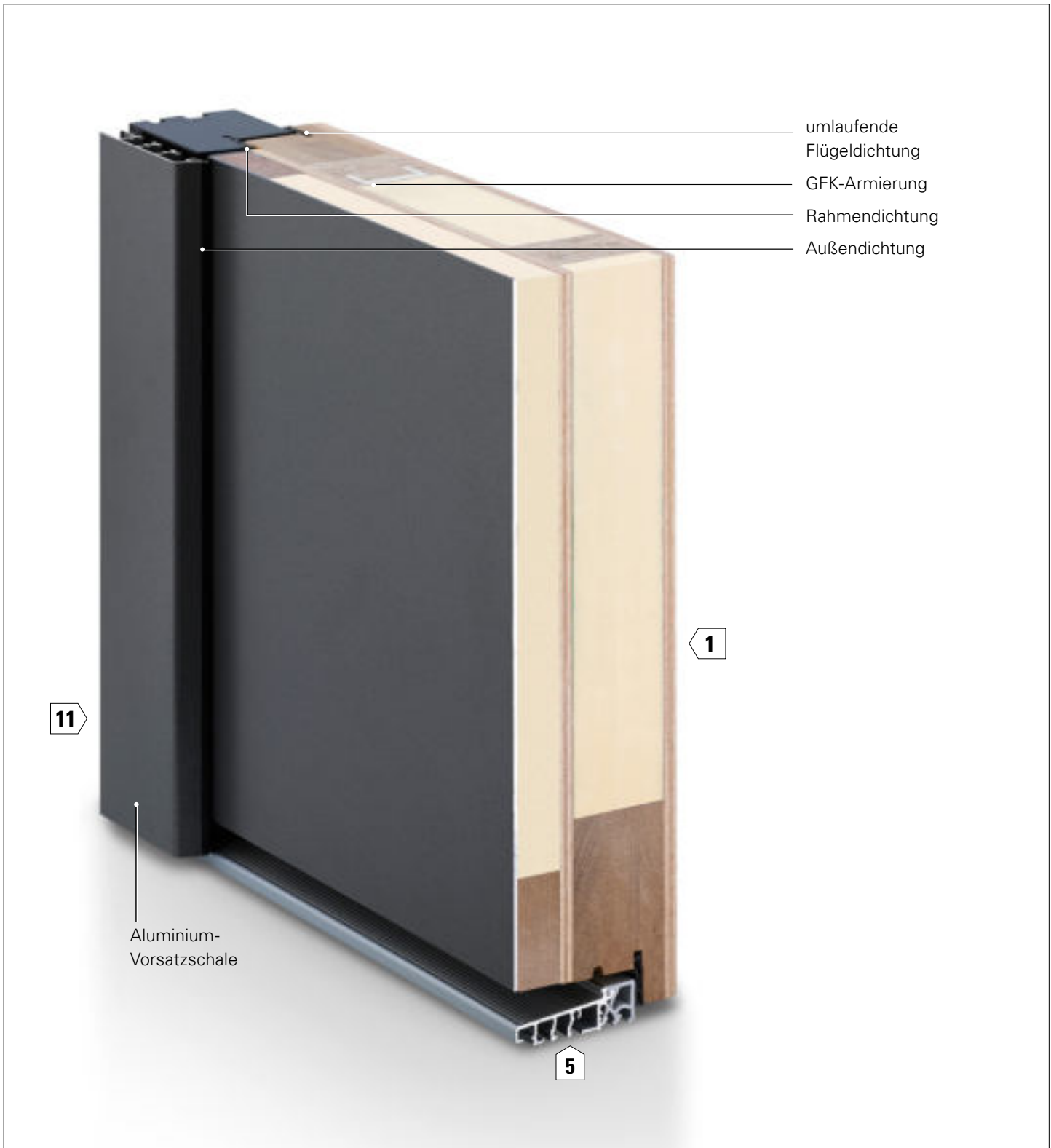
Abb. = Türblattkonstruktion. Fertigungstechnisch bedingt kann auch eine Rahmenkonstruktion erforderlich sein (Bsp. Modell HA H9).
